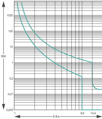
ХАРАКТЕРИСТИКА D
