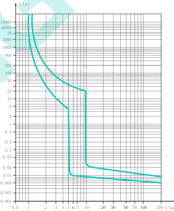
ХАРАКТЕРИСТИКА С
