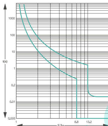
ХАРАКТЕРИСТИКА С
