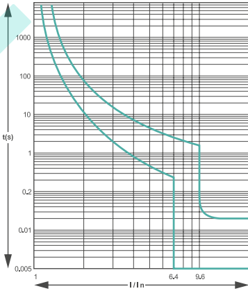
ХАРАКТЕРИСТИКА С
