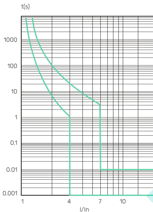
ХАРАКТЕРИСТИКА В
