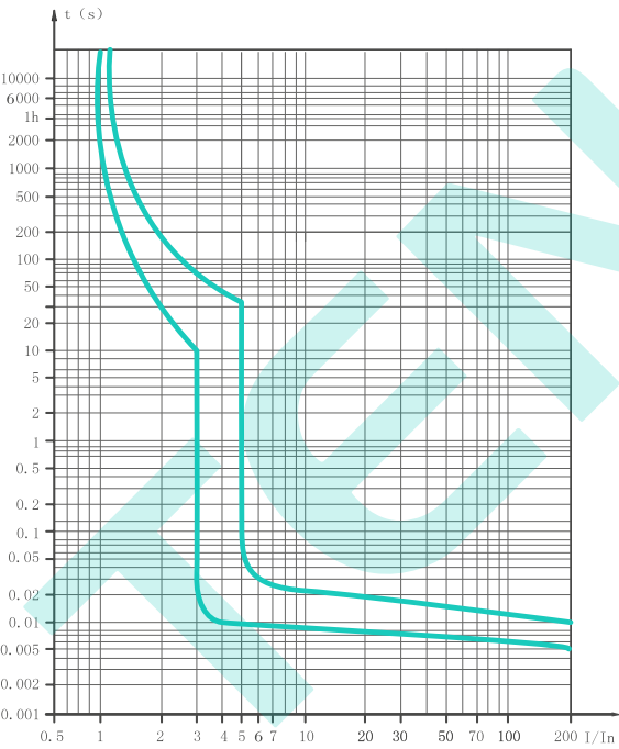
ХАРАКТЕРИСТИКА В
