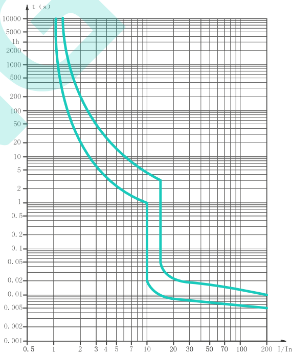
ХАРАКТЕРИСТИКА D
