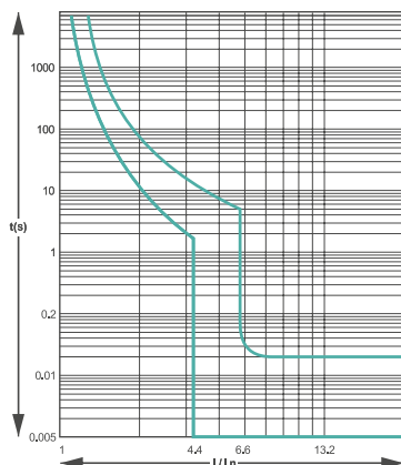
ХАРАКТЕРИСТИКА В
