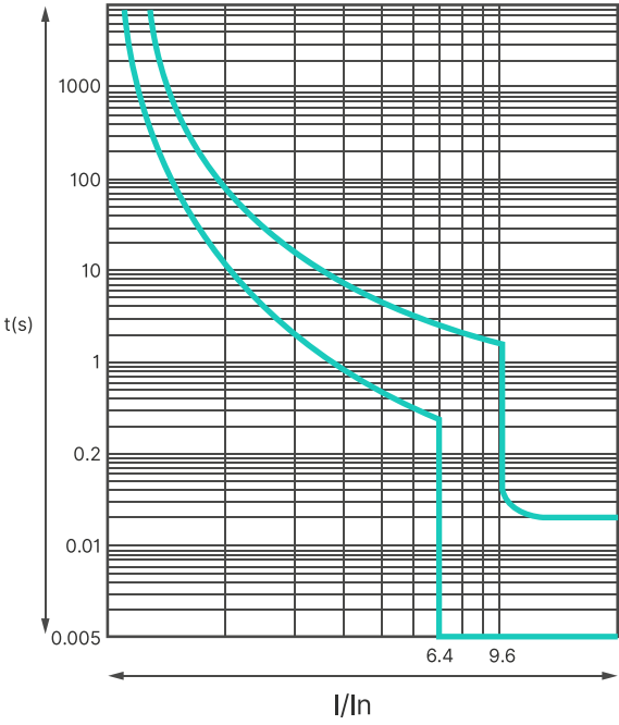
ХАРАКТЕРИСТИКА С
